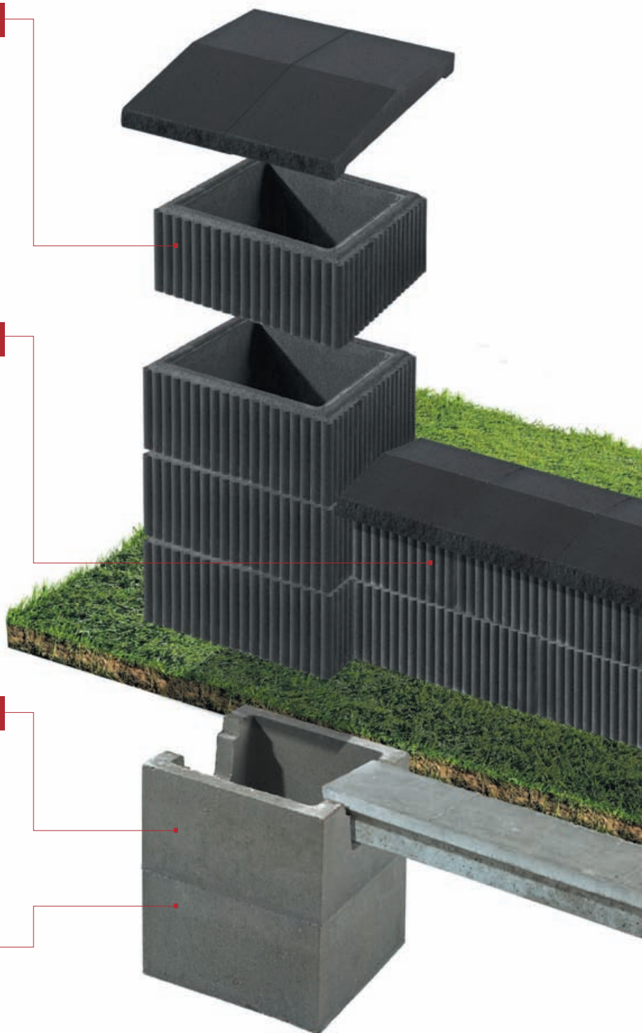
Pustak fundamentowy (z wpustem) symbol: D2 waga: ok. 30 kg
