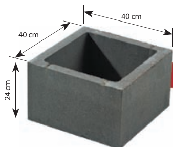
Pustak fundamentowy (pełny) symbol: D1 waga: ok. 33 kg
