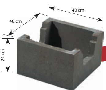
Pustak fundamentowy (z wpustem) symbol: D2 waga: ok. 30 kg
