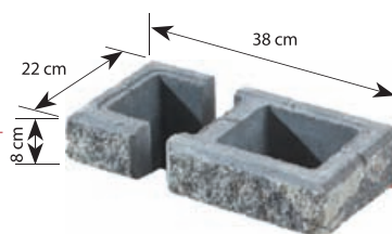
Pustak łupany (słupkowy) symbol: F2 waga: ok. 8 kg
