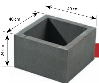
Pustak fundamentowy symbol: D1 waga: ok. 33 kg
