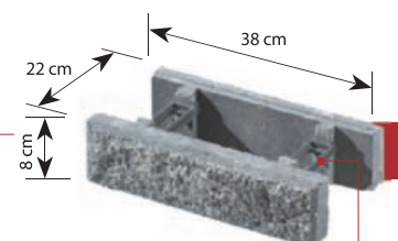
Pustak z kształtek (podmurówkowy) symbol: F3 waga: ok. 6 kg
