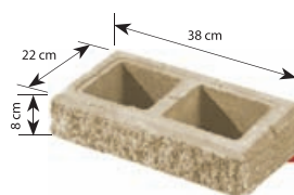
Pustak łupany symbol: A4 waga: ok. 8 kg
