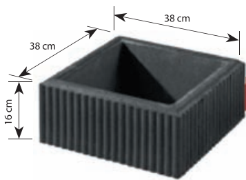
Pustak ryflowany (słupkowy) symbol: C1 waga: ok. 20,5 kg
