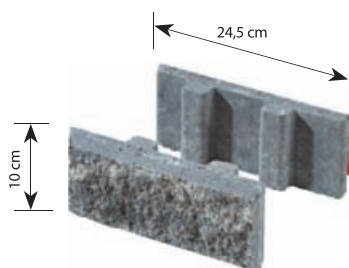
Kształtka łupana prosta symbol J waga: ok. 1,8 kg
