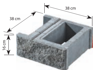
Pustak łupany (podmurówkowy) symbol: B1 waga: ok. 25,5 kg
