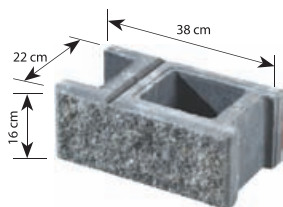
Pustak łupany (podmurówkowy) symbol: A1 waga: ok. 19,2 kg
