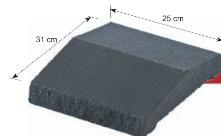
Pustak słupkowy
