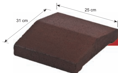
Pustak słupkowy
