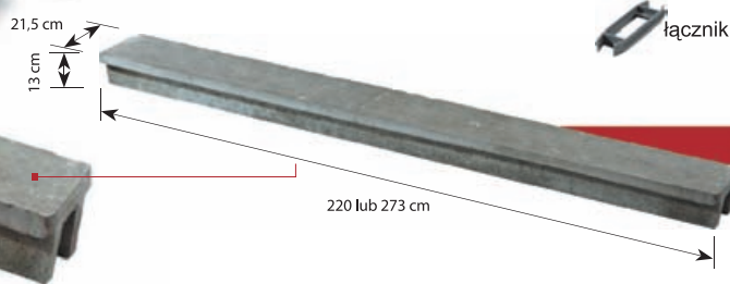
Belka podwalinowa (zbrojona) symbol: D3 (220 cm) waga: ok. 80 kg symbol: D3 (273 cm) waga: ok. 95 kg
