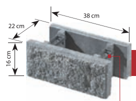
Pustak z kształtek (podmurówkowy) symbol: A3 waga: ok. 12 kg
