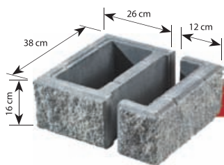
Pustak łupany (słupkowy) symbol: B2 waga: ok. 25,5 kg
