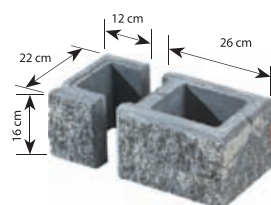
Pustak łupany (słupkowy) symbol: A2 waga: ok. 19,2 kg
