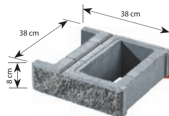
Pustak łupany (podmurówkowy) symbol: G1 waga: ok. 13 kg
