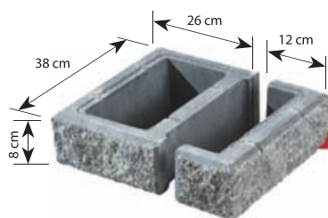
Pustak łupany (słupkowy) symbol: G2 waga: ok. 13 kg
