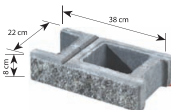
Pustak łupany (podmurówkowy) symbol: F1 waga: ok. 8 kg
